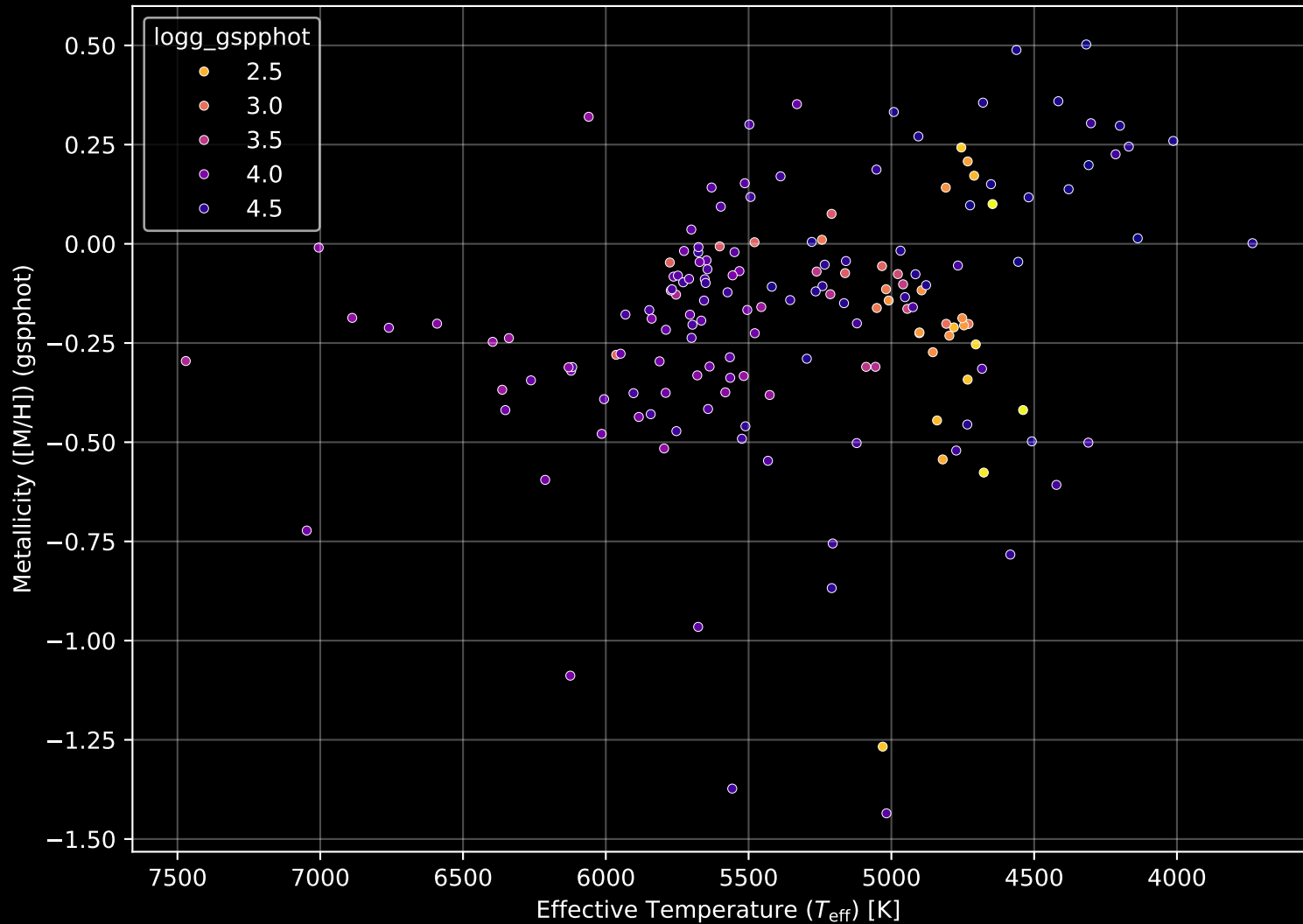
APOGEE DR17 Field: [048+41_MGA] Stellar Population Parameters (n= 166)
